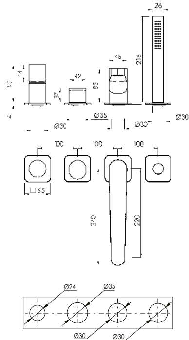
mm Agujeros de instalación Installation holes Perçages d'installation
